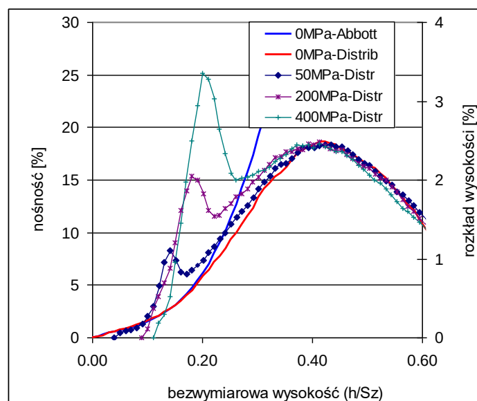
Rys. 5.4 Powiększony początkowy fragment rozkładów wysokości powierzchni z rys. 5.3
