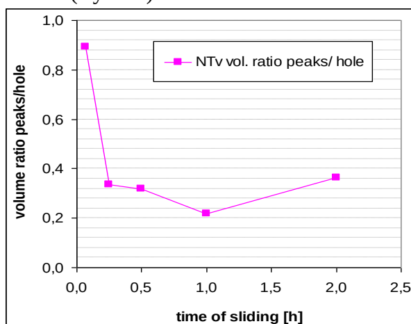
Rys. 6.4. Stosunek objętości wypływek (peaks) do rowku zużycia (hole) w funkcji czasu zużycia (NiTi austenit)
