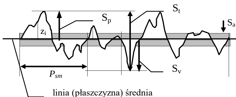
Rys. 2.3 Schemat profilu z wybranymi parametrami
