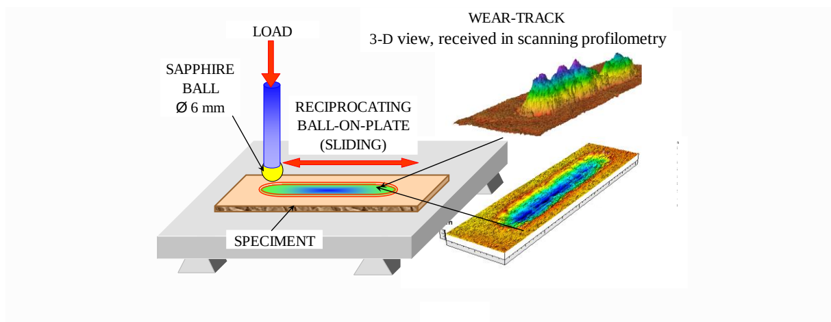
Rys.6.1. Schemat urządzenia do badania zużycia i graficzna ilustracja wyznaczenia metodą profilometryczną objętości ubytku materiału podczas „dry-sliding” testu.
