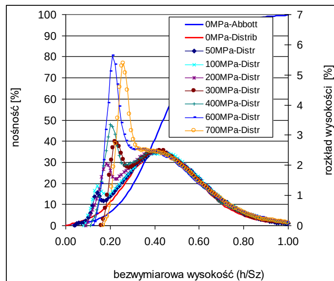
Rys.5.3 Porównanie przebiegów rozkładów wysokości dla powierzchni piaskowanej obciążanych do różnych wartości naprężenia
