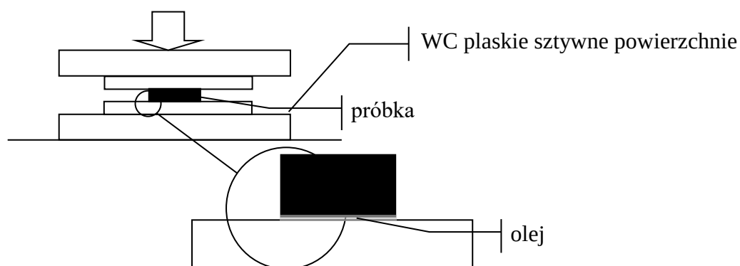
Rys. 3.2 Schemat obciążania kontaktowego próbki
