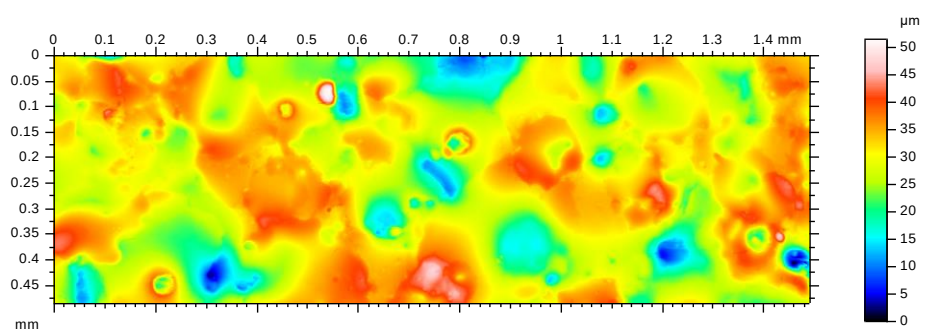
Rys. 4.1a Struktura powierzchni przed obciążeniem.
