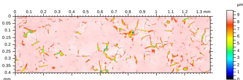
Rys. 4.1d Struktura powierzchni po odkształceniu 34% bez oleju.
